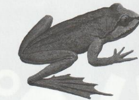
Hyogobatrachus wadai
